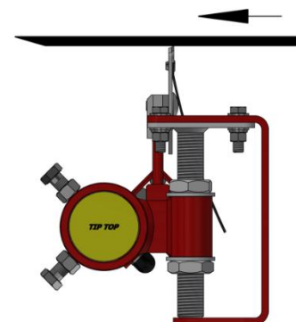
Einbau REMACLEAN HM-U10 S
