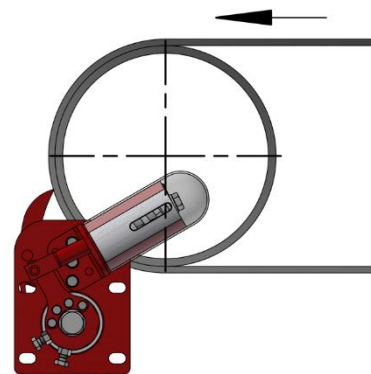
Einbau REMACLEAN PUR-F5
