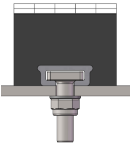
REMASLIDE ALOX Querschnitt
