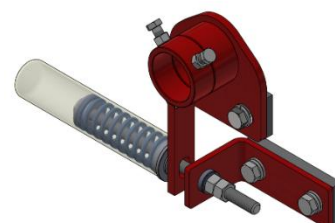
PUR-F6 Spannvorrichtung V2, Spannseite
