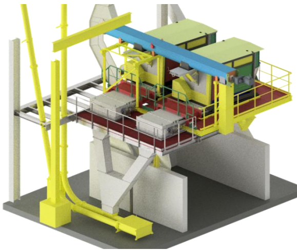
Erweiterung Siebanlage
