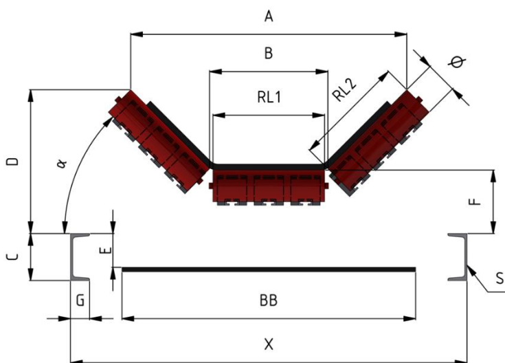
Maßangaben zur kundenspezifischen Fertigung
