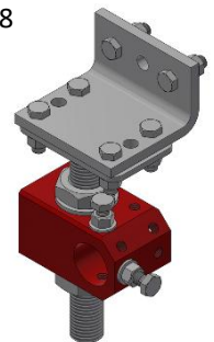
Anpressvorrichtung HM-U7
