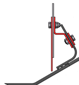
REMASKIRT CB 195 mit Montageschiene
