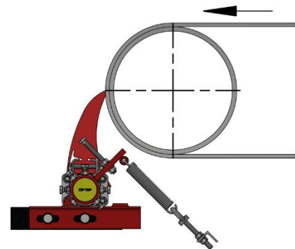
Einbau REMACLEAN PUR-F4
