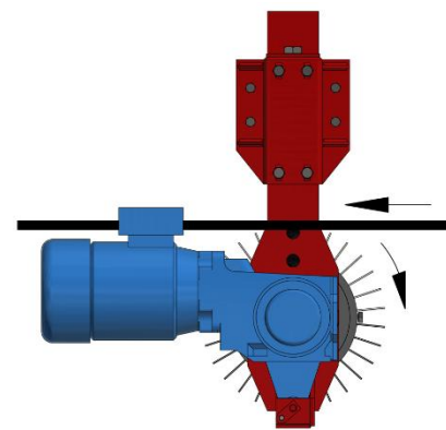
Einbau REMACLEAN GBM
