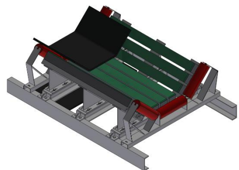
Prallbalkentisch inkl. Prallbalken
