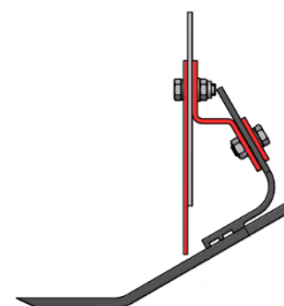
REMASKIRT CB 195 mit Montageschiene
