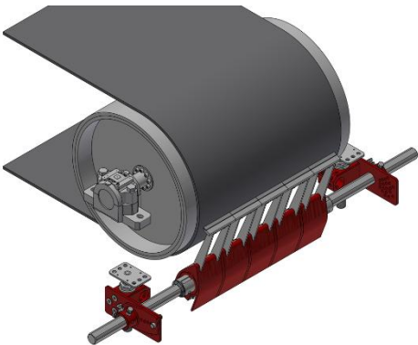
Einbau LSPV V1
