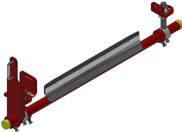
Einbau Abklappvorrichtung
