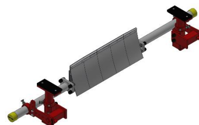
Stufenplatte HM-U1/U2
