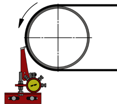
Einbau REMACLEAN HM-F2
