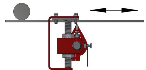
Einbau REMACLEAN HM-U11R
