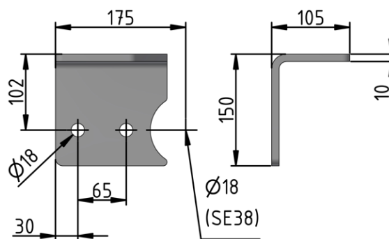
Spanneinheit für \square 67 mm (SE38)
