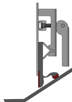
Einbau inkl. Klemmsystem
