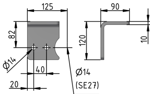
Spanneinheit für \square 52 mm (SE27)
