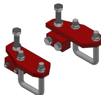
Reversieranschlag HM-U1/U2
