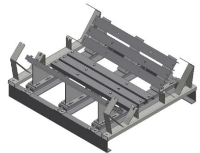
Stahlkonstruktion - Prallbalkentisch
